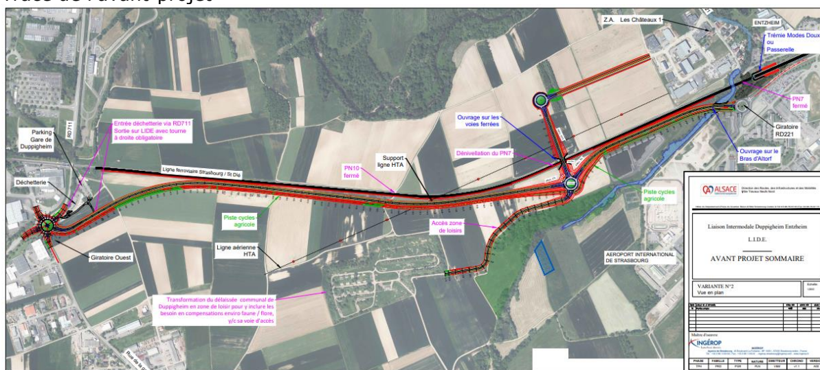
Tracé de l'avant-projet
