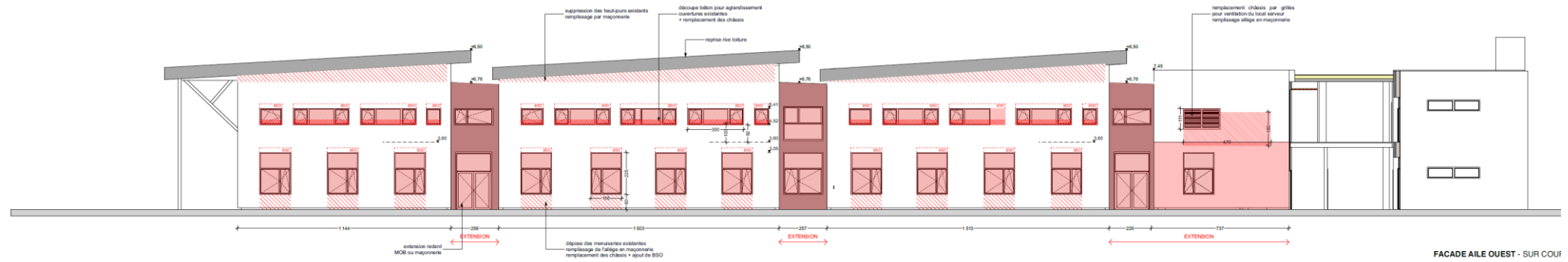
FACADE AILE OUEST - SUR COUI
