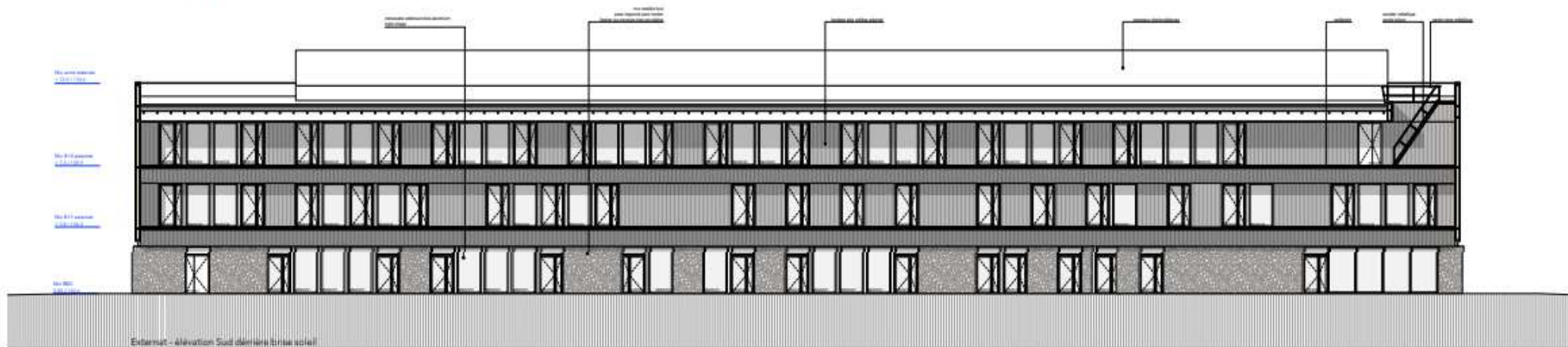
Façade SUD derrière les brises soleil
