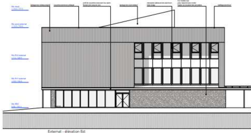
Façade EST
