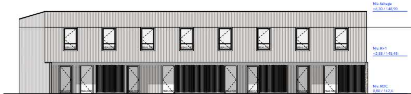
Logements - élévation Ouest
