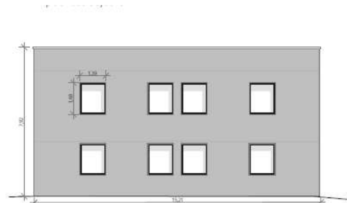
FACADE NORD-EST V1 - LOGEMENTS
