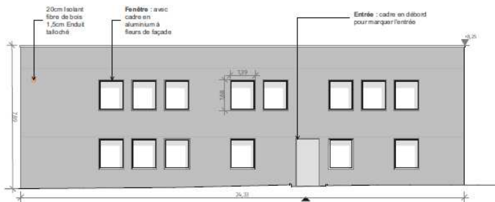
FACADE NORD-OUEST V1 - LOGEMENTS
