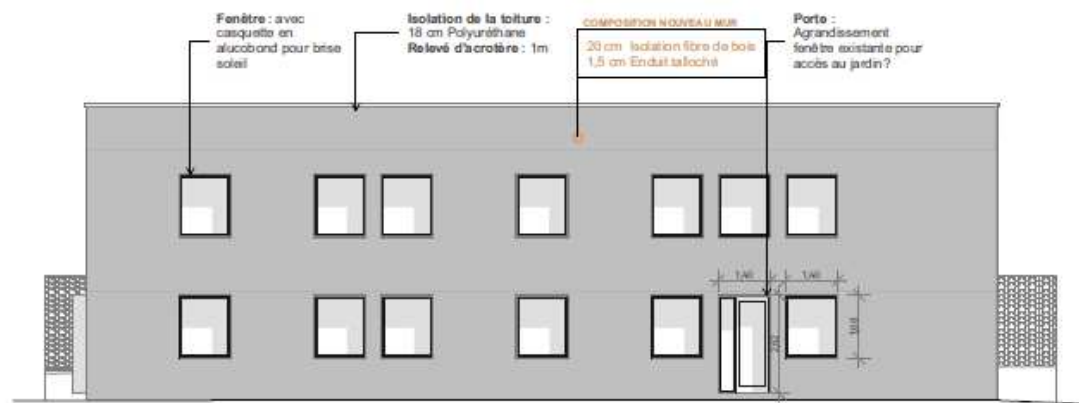
FACADE SUD-EST V1 - LOGEMENTS
