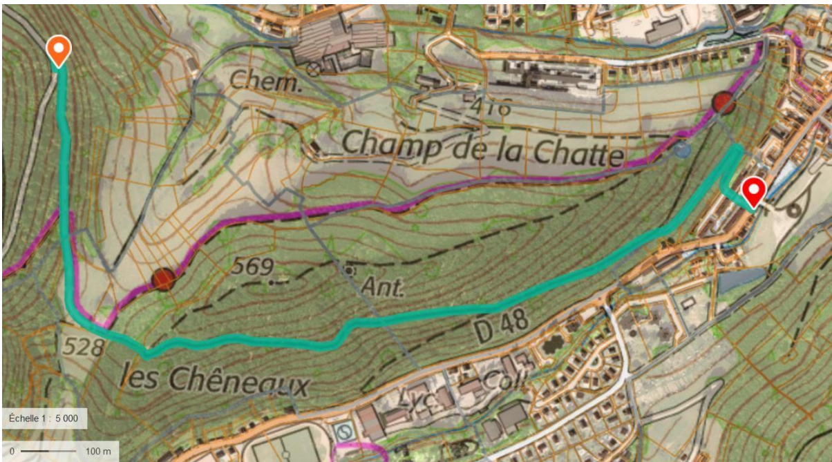
Plan de détail chemin du Saegerthal
