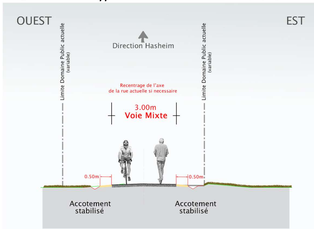
Profil en travers type Rue de Sainte Barbe à SCHLIERBACH
