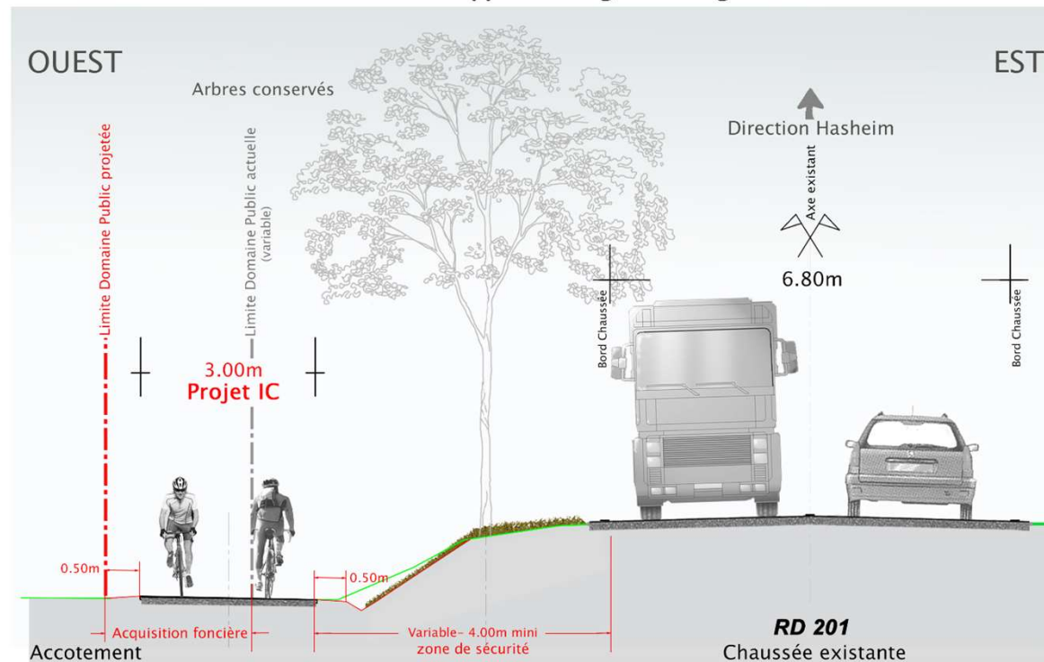
Profil en travers type le long de l'alignement d'arbres
