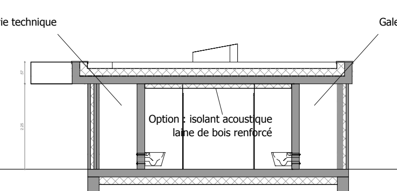
Bloc sanitaires élèves - Coupe transversale ech :1/100
