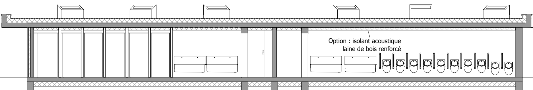
Bloc sanitaires élèves - Coupe longitudinale ech :1/100
