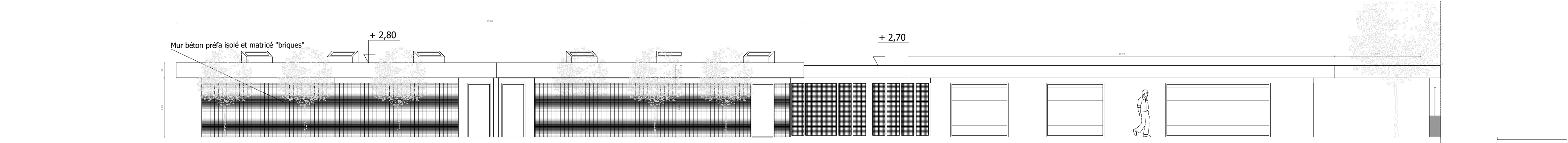
Bloc sanitaires élèves - Façade Nord et bloc garages existant ech :1/100
