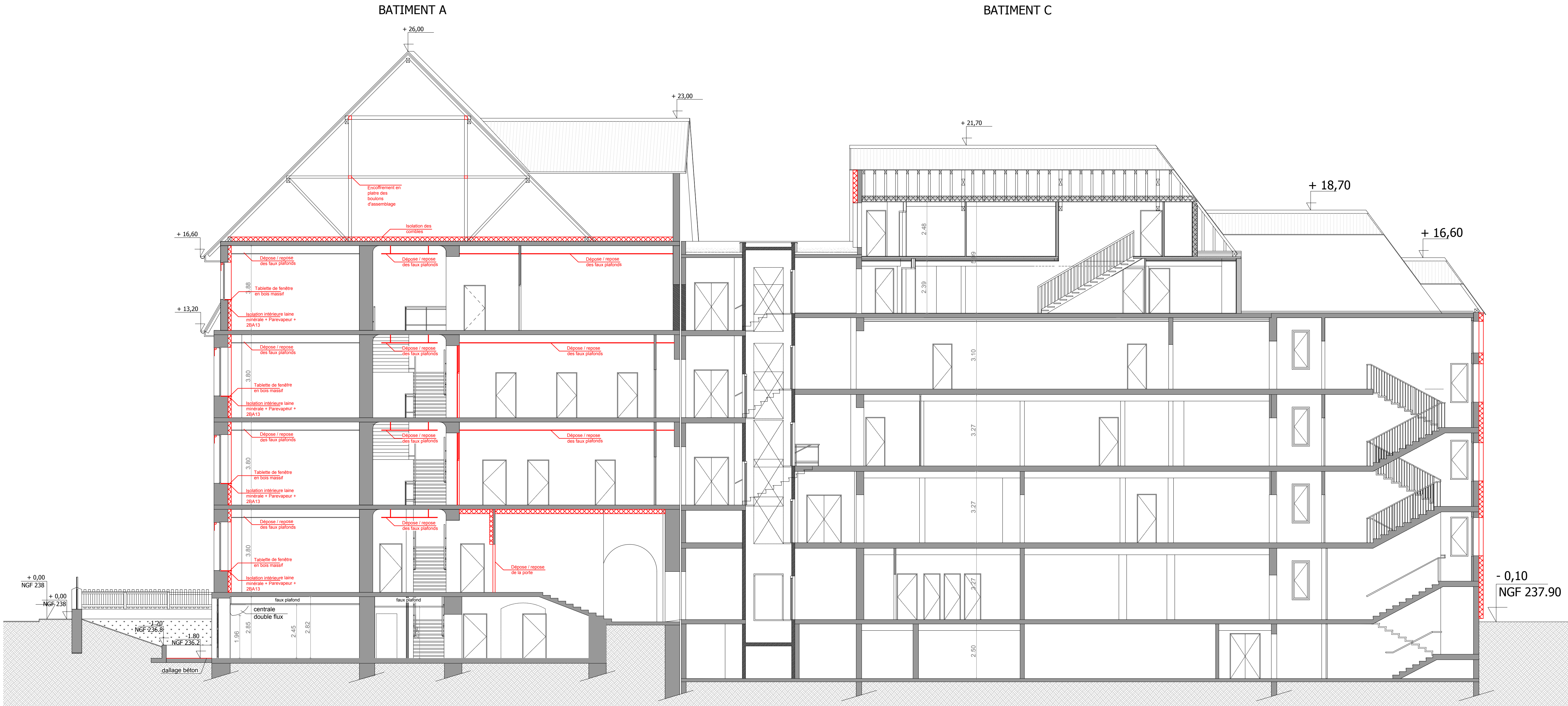
Coupe transversale AA ech :1/100
