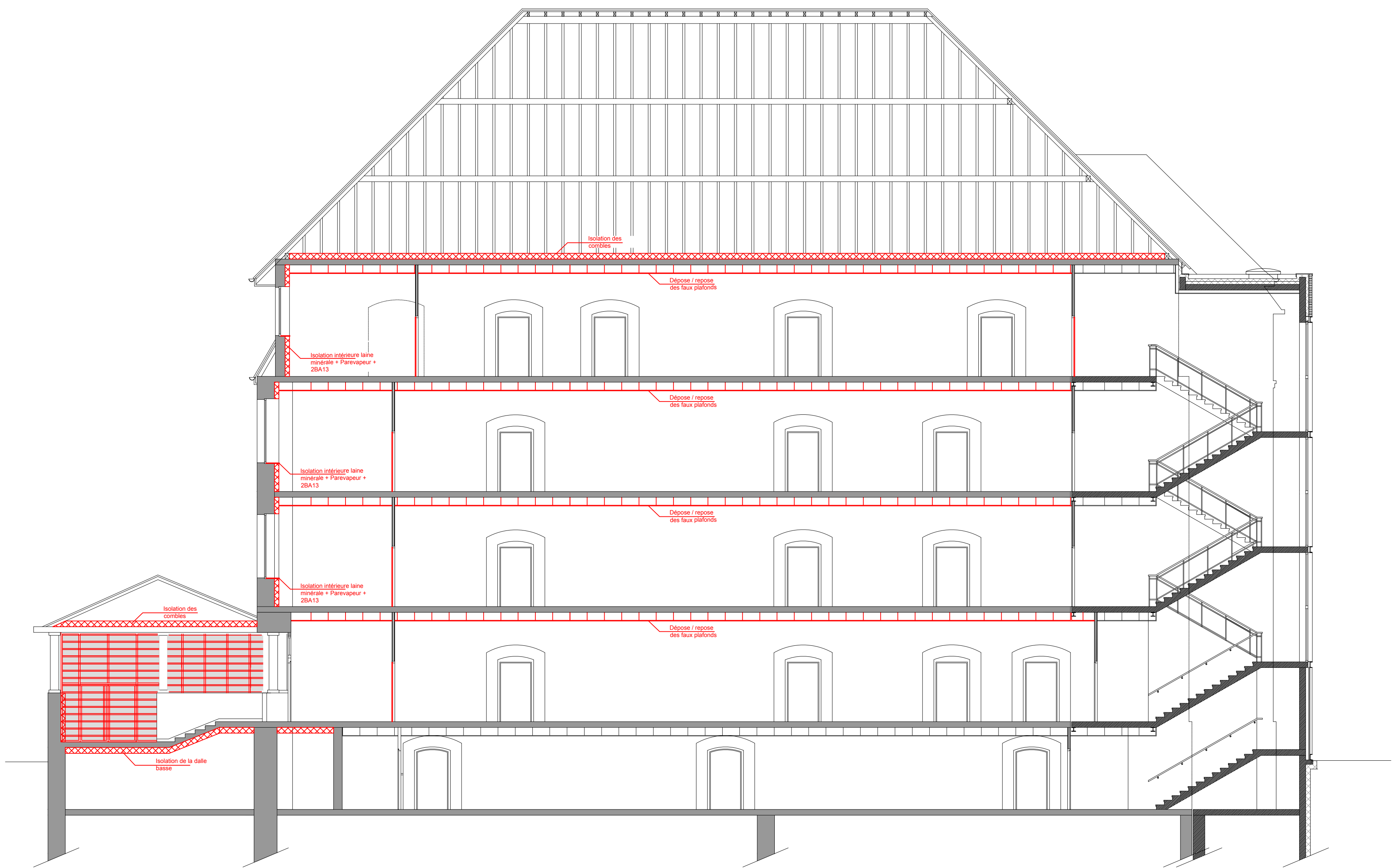
Coupe longitudinale BB ech :1/100
