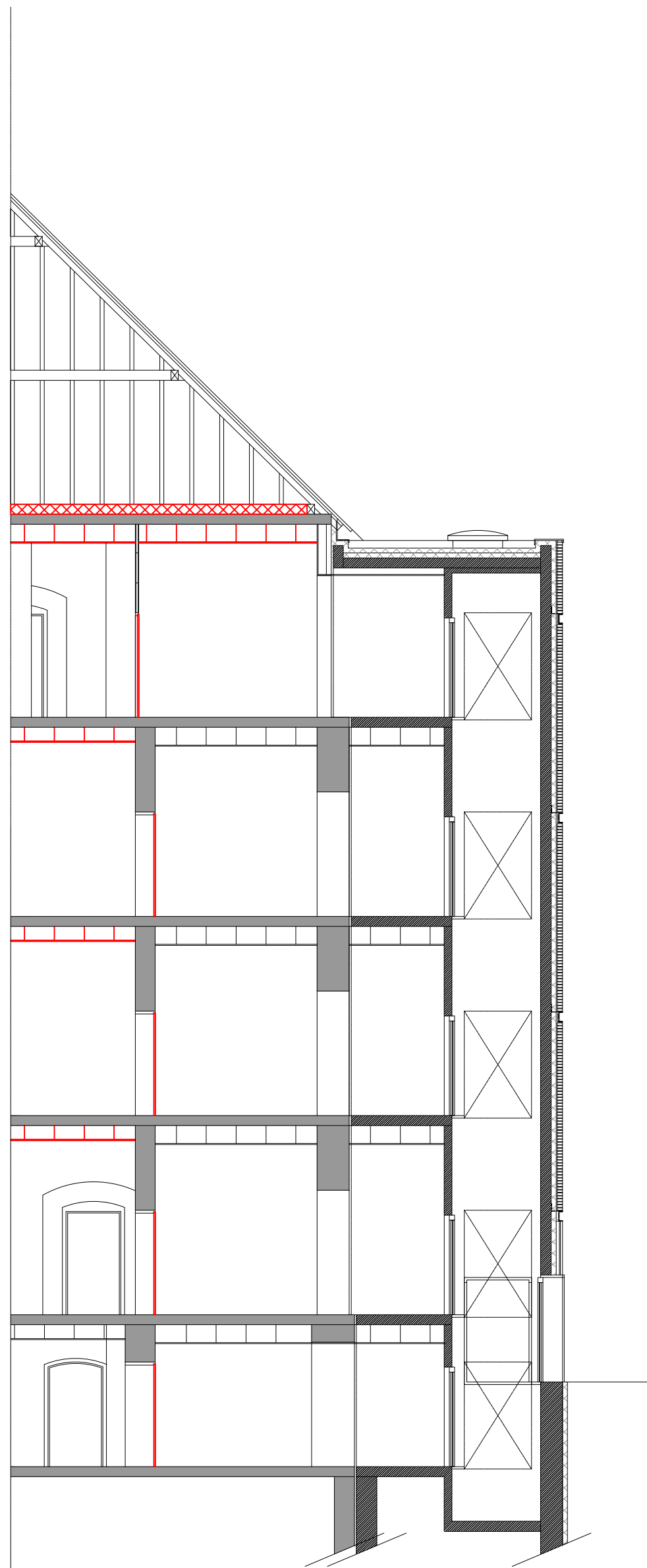
Coupe longitudinale B'B' ech :1/100
