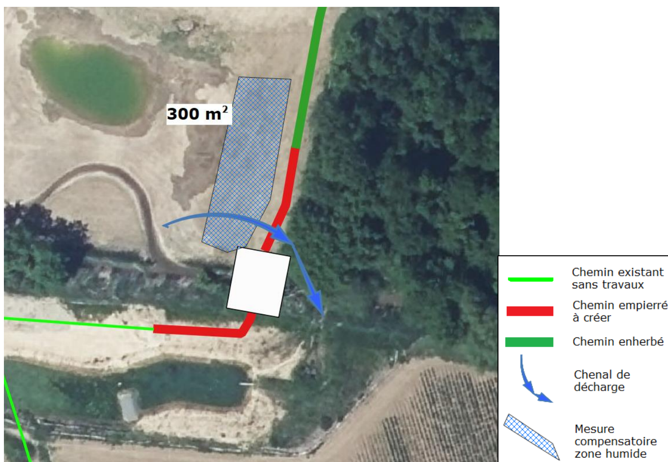
Fig. 36. Pont n°5 sur le MUEHLBACH à BREUSCHWICKERSHEIM : chenal de décharge en rive gauche (présence de réseau en rive droite) et mesure compensatoire ZH de 300 m 2
