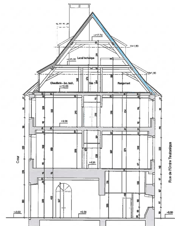
COUPE BB sur l'entrée Sud
