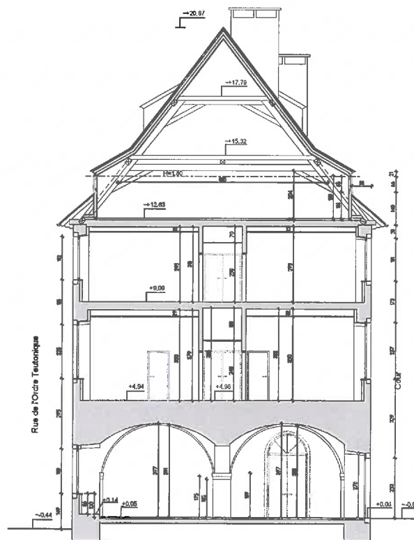
COUPE AA sur la salle d'expositions
