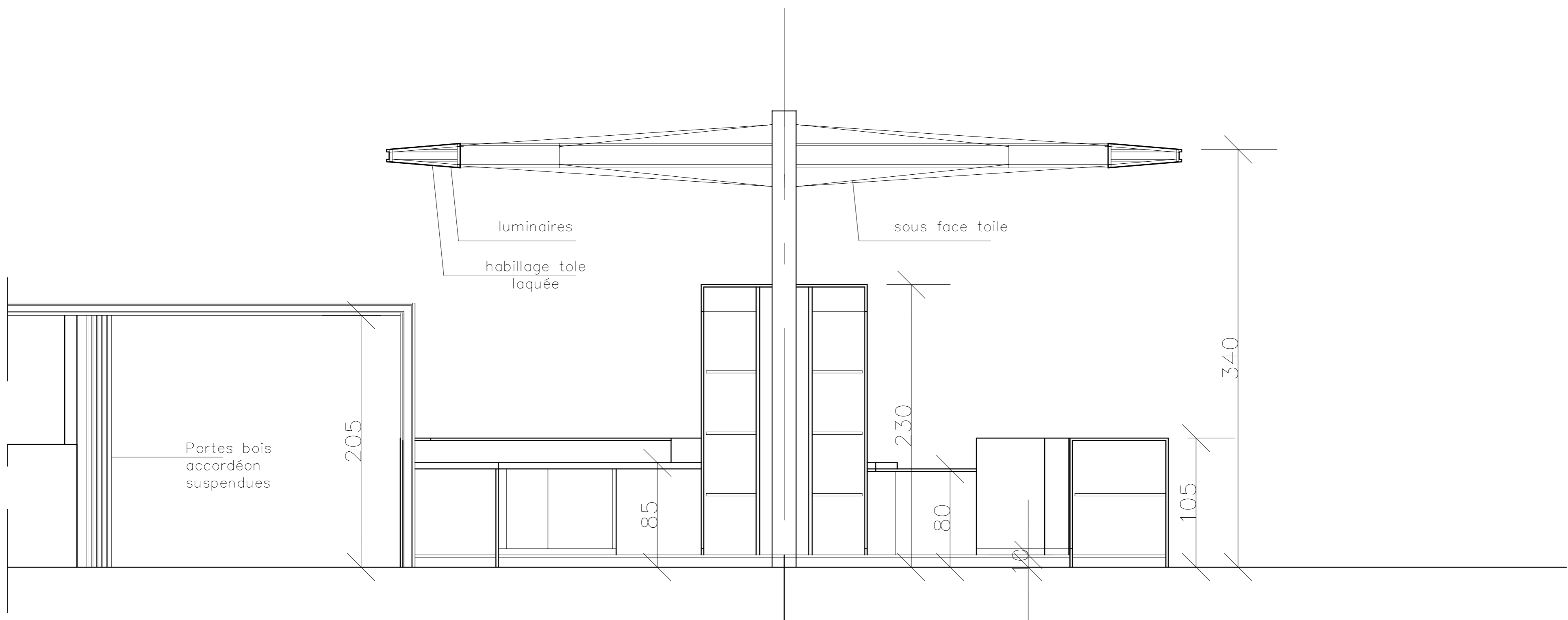
COUPE A-A
